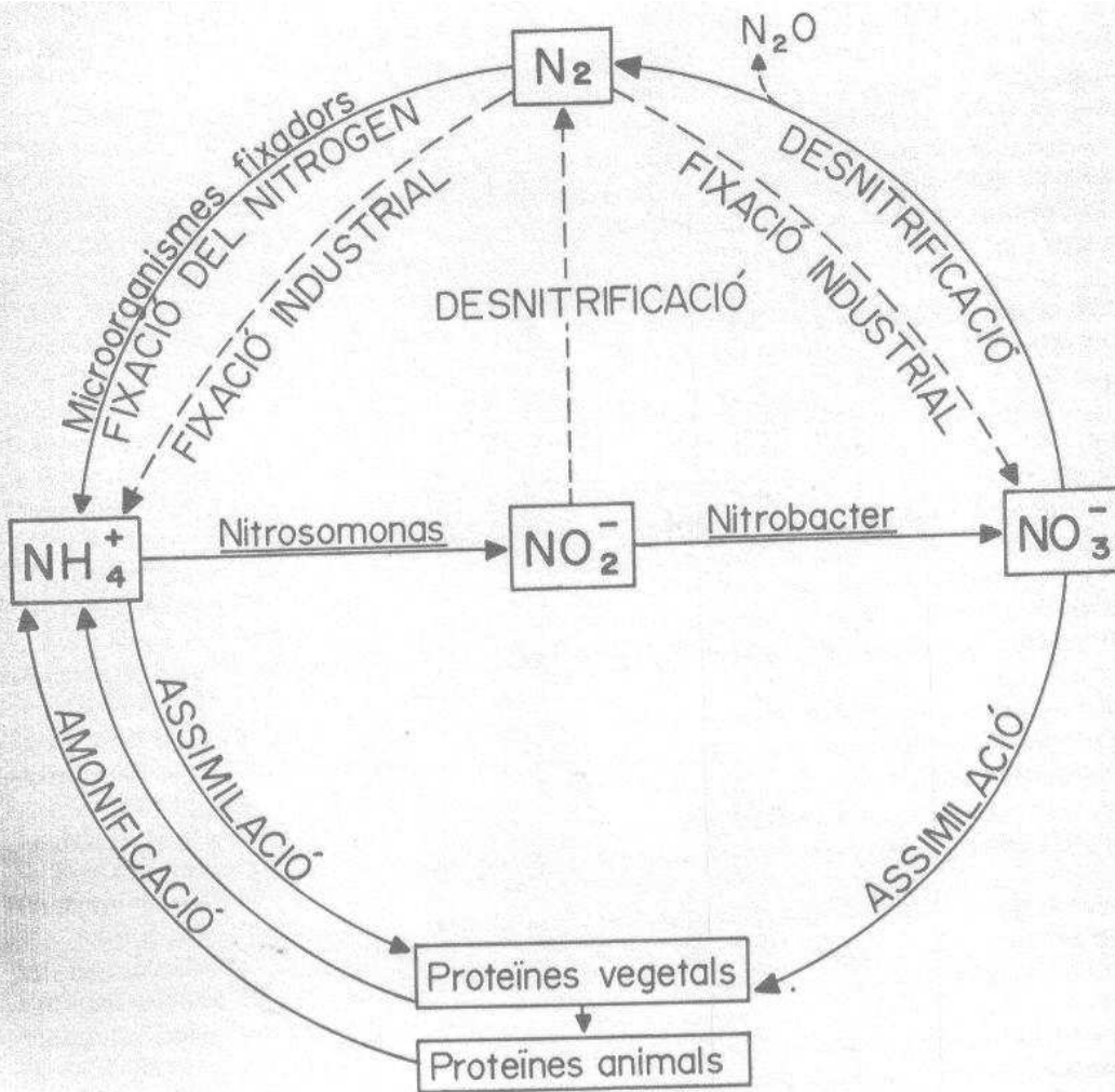
FIGURA 13. El cicle del nitrogen.
