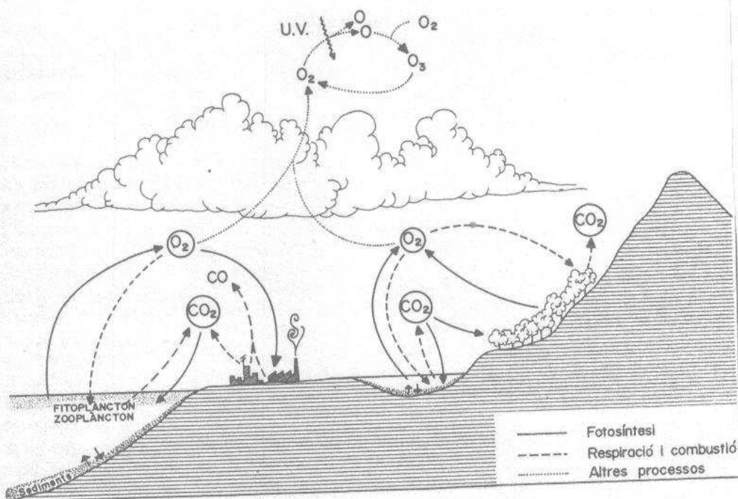
FIGURA 14. El cicle de l'oxigen.
